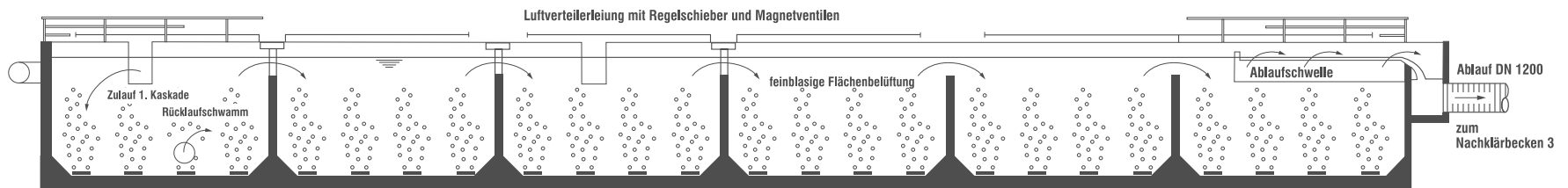
Schnitt A-A:
